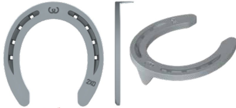
Toe clip
